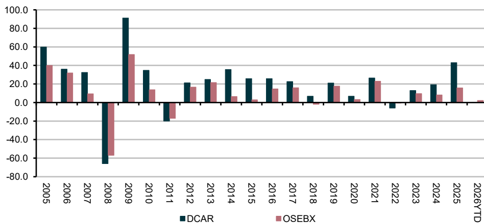
Figure 3: Historisk porteføljeavkastning, 2005-2026
