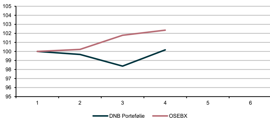
Figure 2: Porteføljeavkastning
